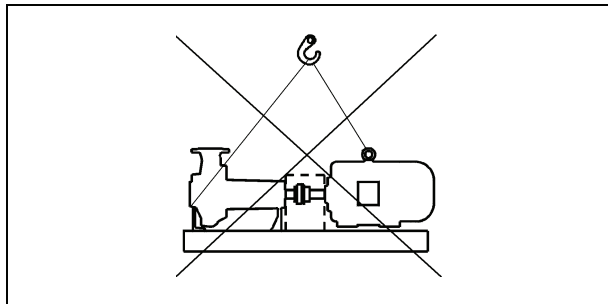
Falscher Transport
