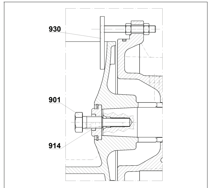
Skizze zur Demontage des Laufrades
