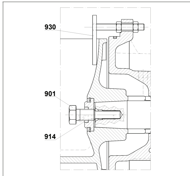
Croquis démontage de la roue
